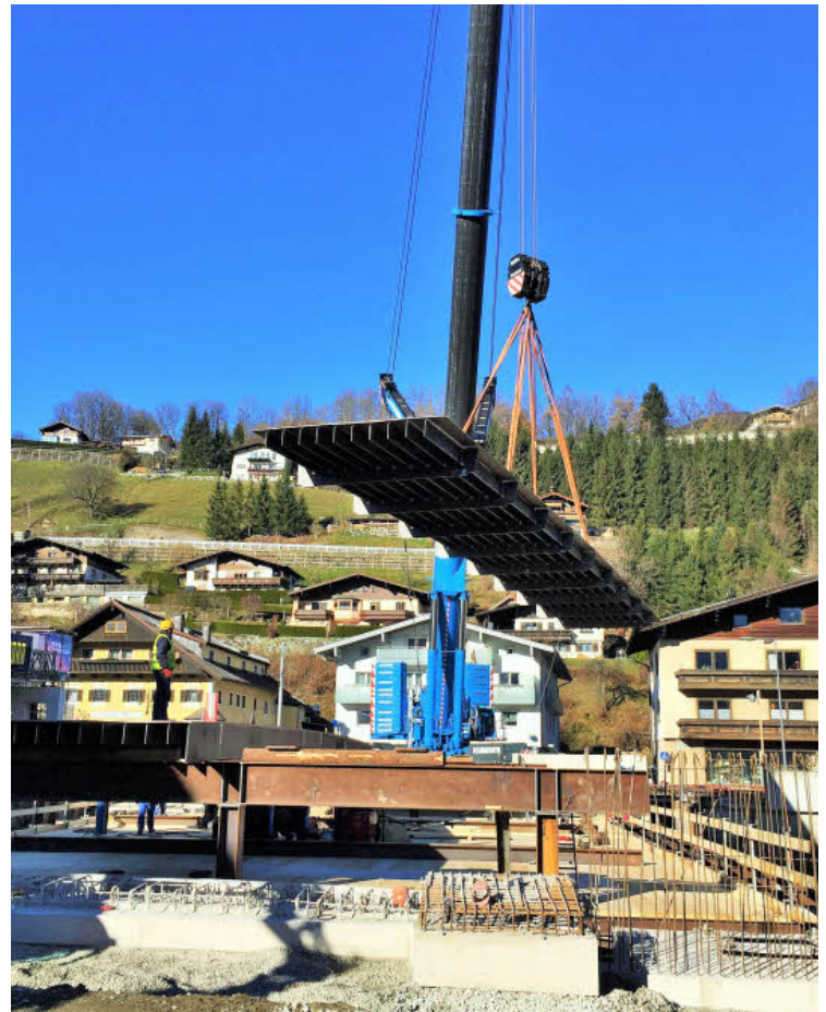
Projektleiter Wolfgang Mariacher vor der im Endausbau 240 Tonnen schweren Stahlbrücke. Rechts: Vorige Woche wurden die Einzelteile – im Bild ein Teil der Fahrbahn – von einem riesigen Autokran eingehoben.
